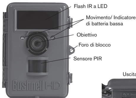
Fig. 1: Connessioni
